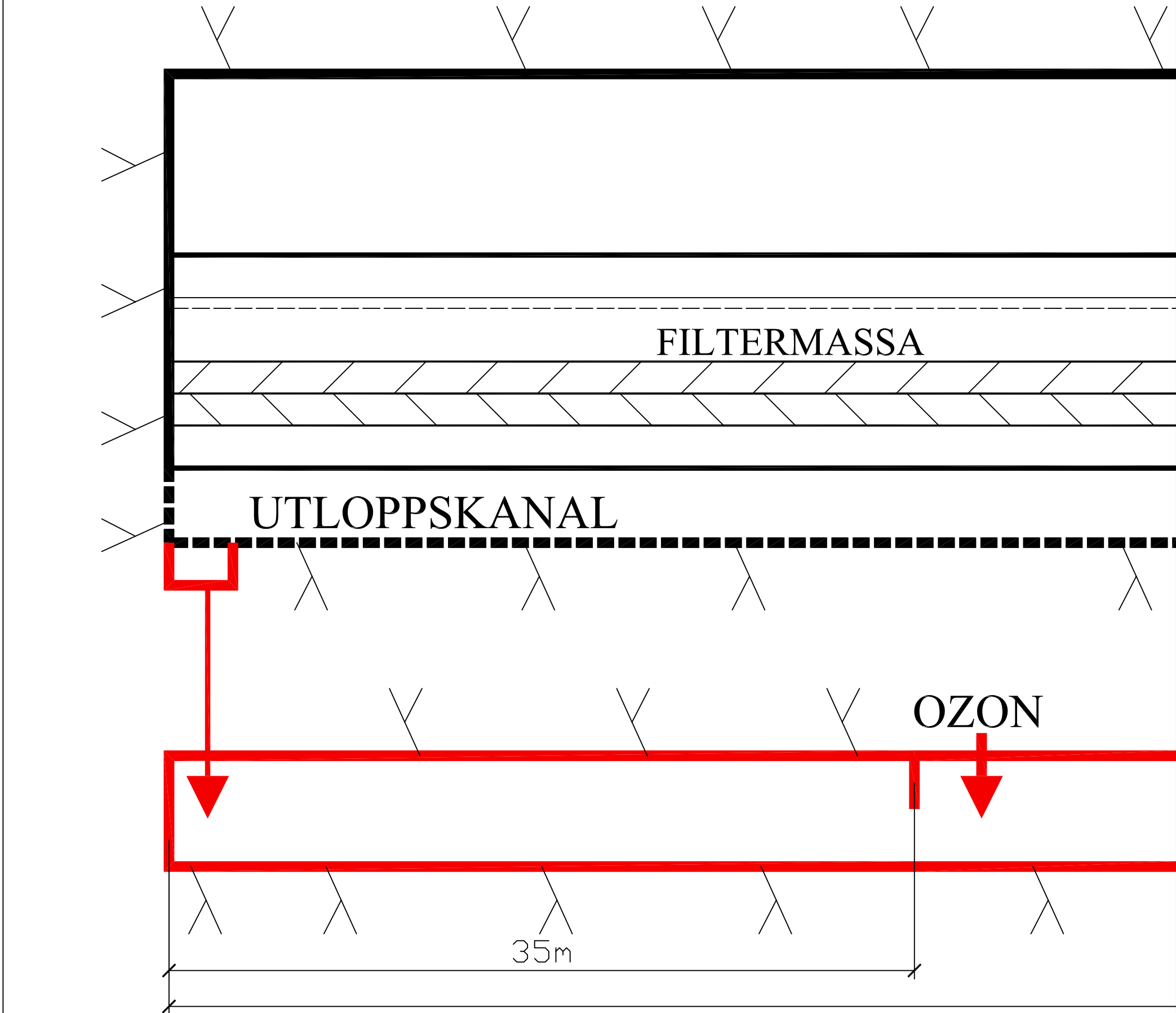
SEKTION A-A
